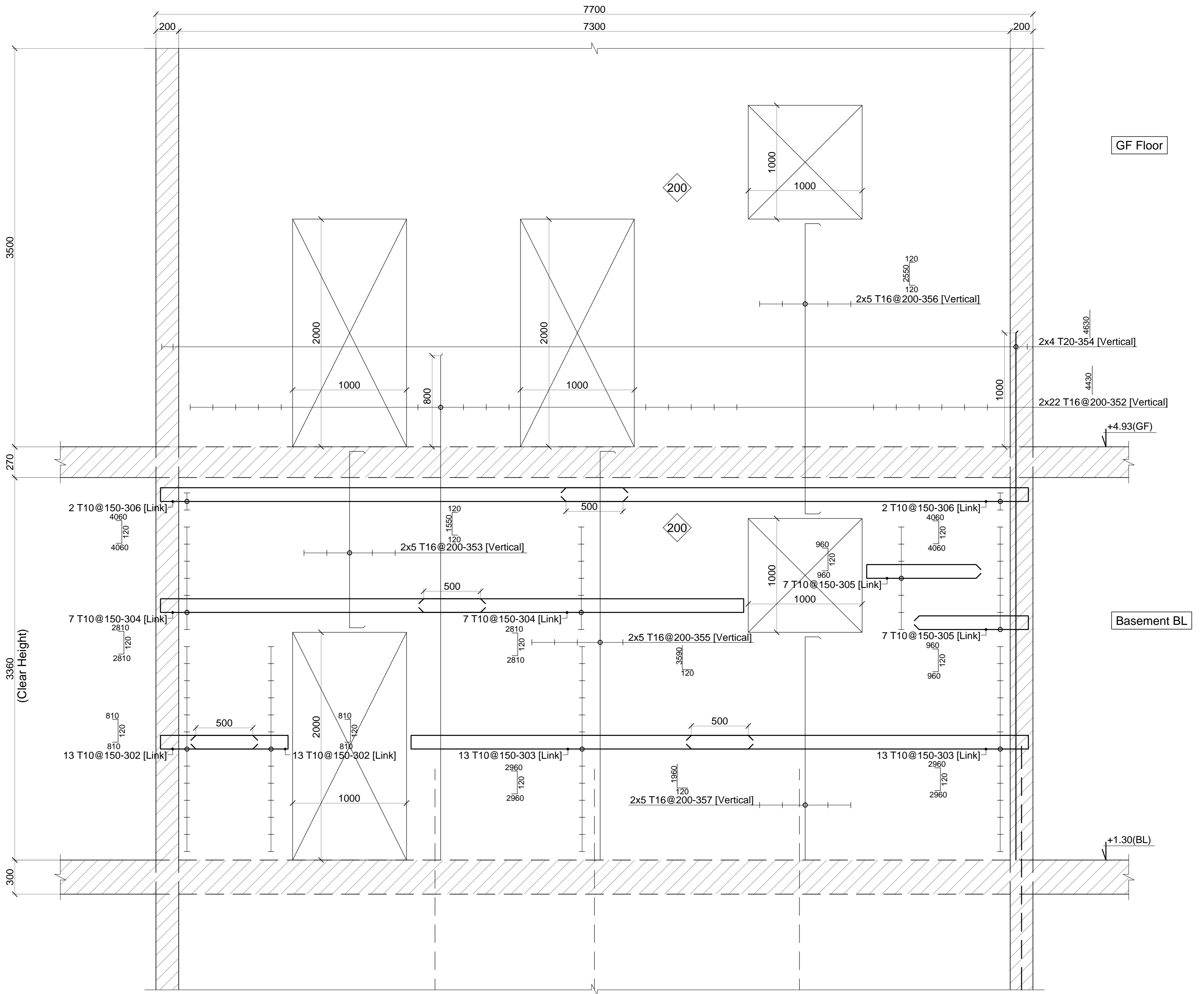
Section 1-1 Scale: 1/25
